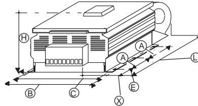
FORI di FISSAGGIO/FIXING HOLES - 4MA screws (470/2-> 470/6,5) - 5MA screws (470/6-> 470/9,5)
